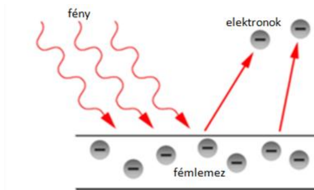
5.ábra A külső fényelektromos hatás
